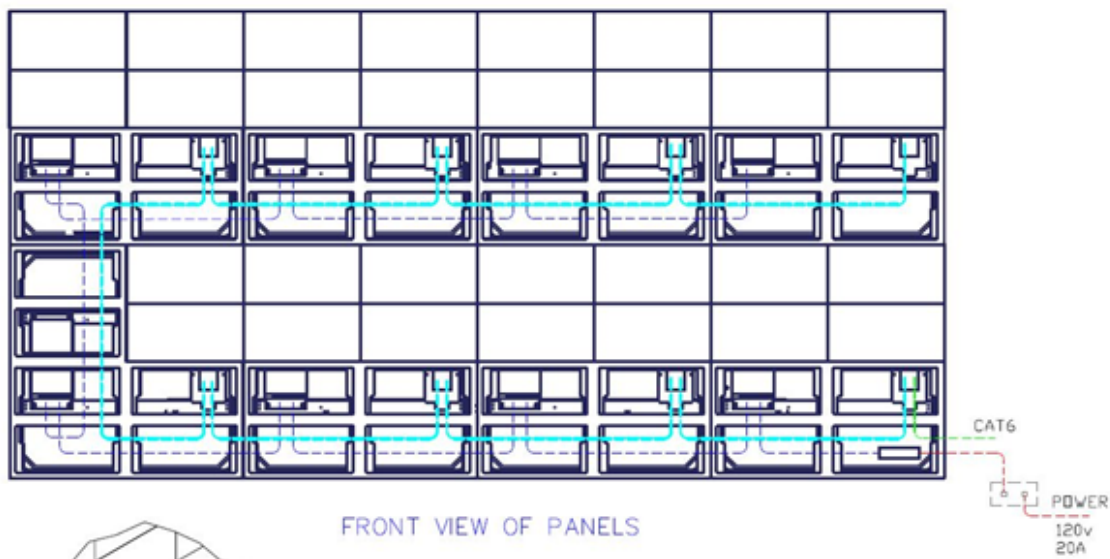
(8810 Wiring Diagram)
