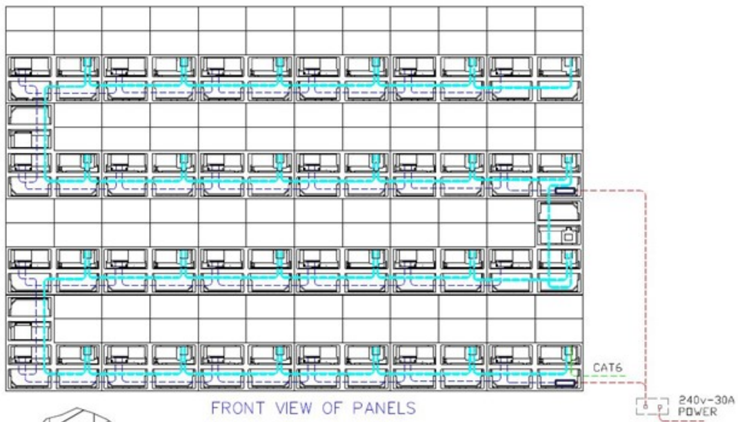
(8830 Wiring Diagram)
